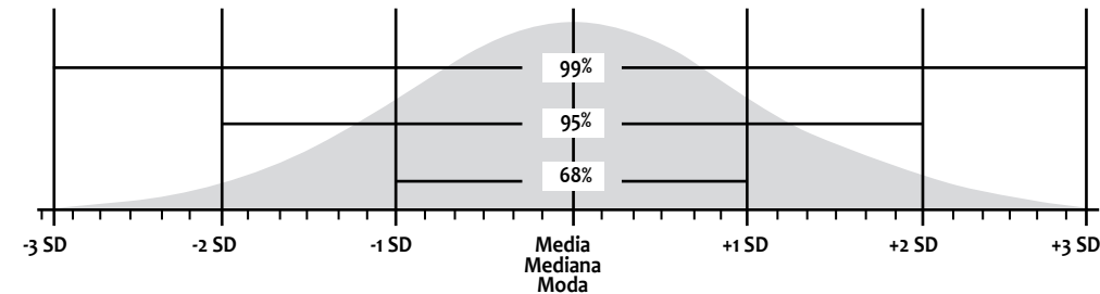
Figura 4-2: Una distribución normal
